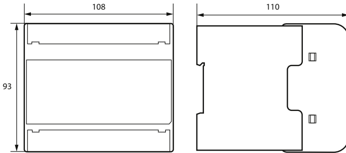
Abbildung: Gehäuse iso685...-Gerätefamilie – Maßangaben in mm
