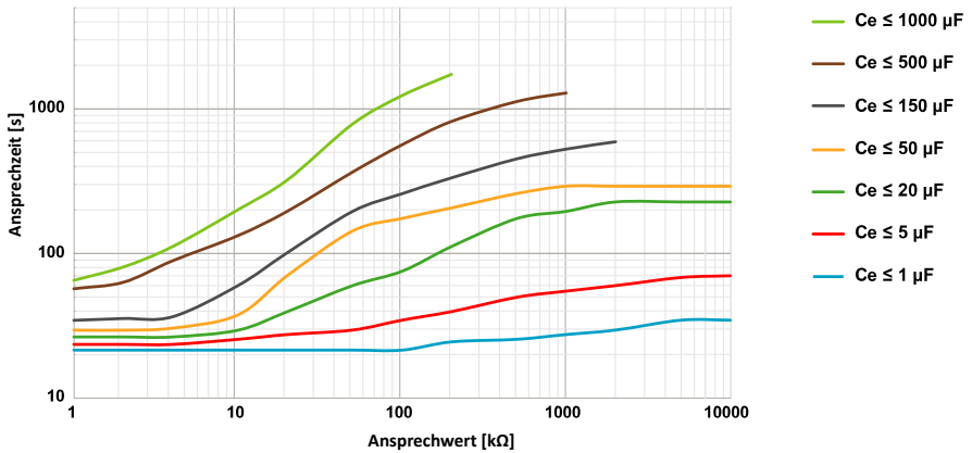
Ansprechzeit t_{an} Profil „Hohe Kapazität“ in Abhängigkeit von Ansprechwert R_{an} und Netzableitkapazität C_e nach IEC 61557-8 ( U_n = 690 V, f = 50 Hz); Messbereich < 10 M \Omega
